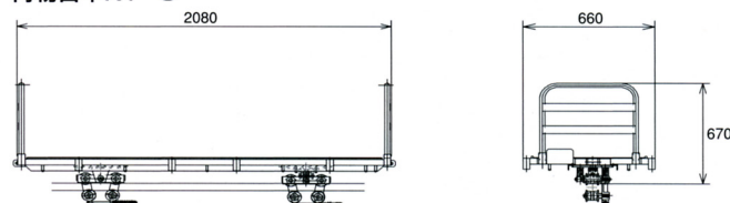
バケット台車(DB-15)
