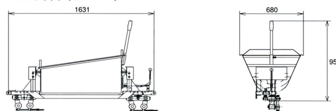
乗用台車KRT-1+荷物台車KT-2
