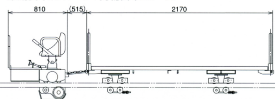
乗用台車KRT-1+荷物台車KT-2
