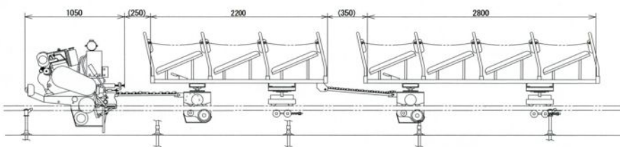
【2】台車の仕様及び構造及び諸元
