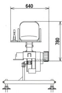
動力車 KS-90NT+乗用台車KRT-3B+乗用台車KRT-4B
