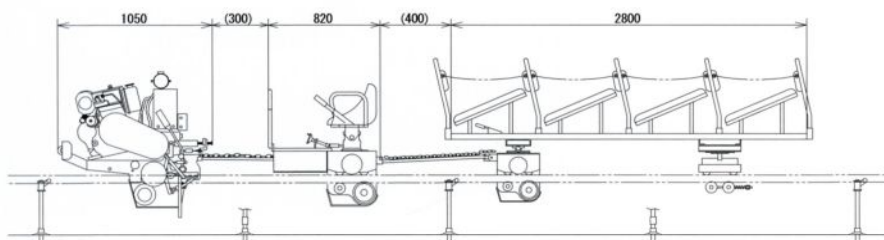
【1】動力車の仕様及び構造・諸元
