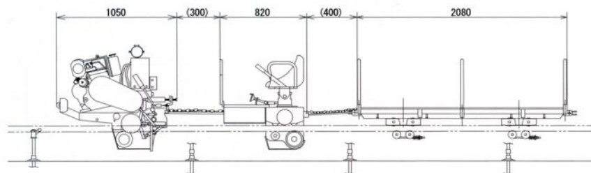
動力車 KS-90NT+乗用台車KRT-1B+乗用台車KRT-4B
